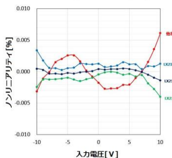
非直線性(ノンリニアリティ)[%] 3σデータ (回帰直線との差)/フルスケール(20V)×100
